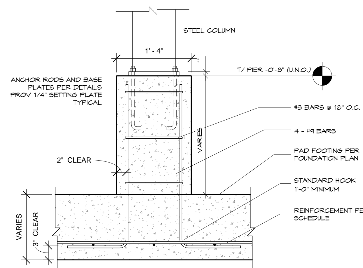
8 Pier - Typ 1" = 1'-0"
