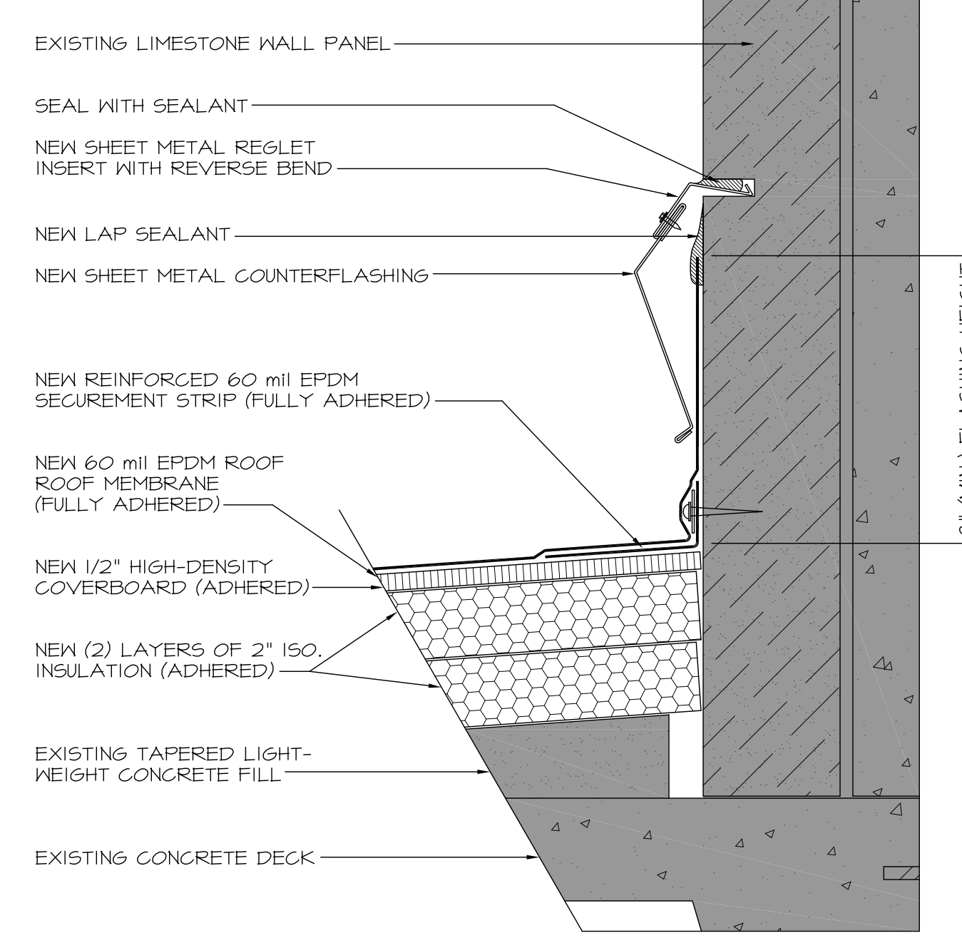
5 WALL FLASHING DETAIL 2 SCALE: 3"=1'-0"
