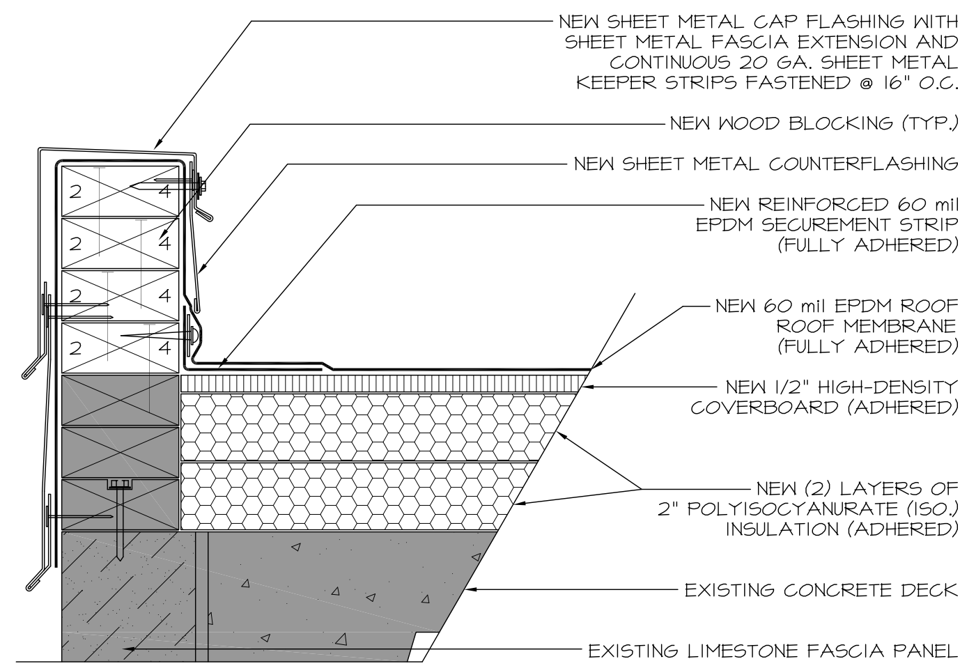
1 EDGE FLASHING DETAIL SCALE: 3"=1'-0"
