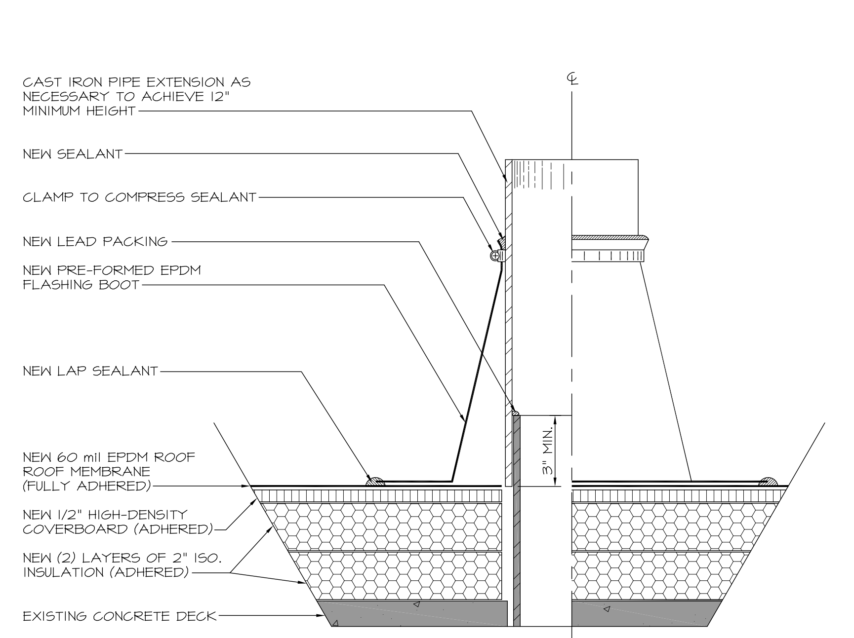
9 PLUMBING VENT DETAIL 2 SCALE: 3"=1'-0"
