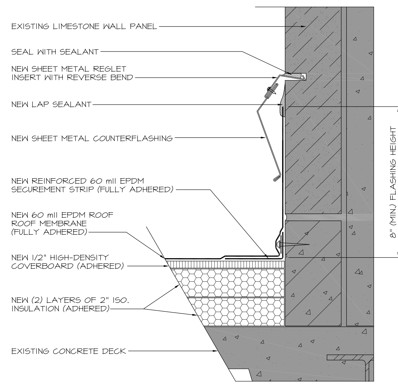
3 WALL FLASHING DETAIL 2 SCALE: 3"=1'-0"
