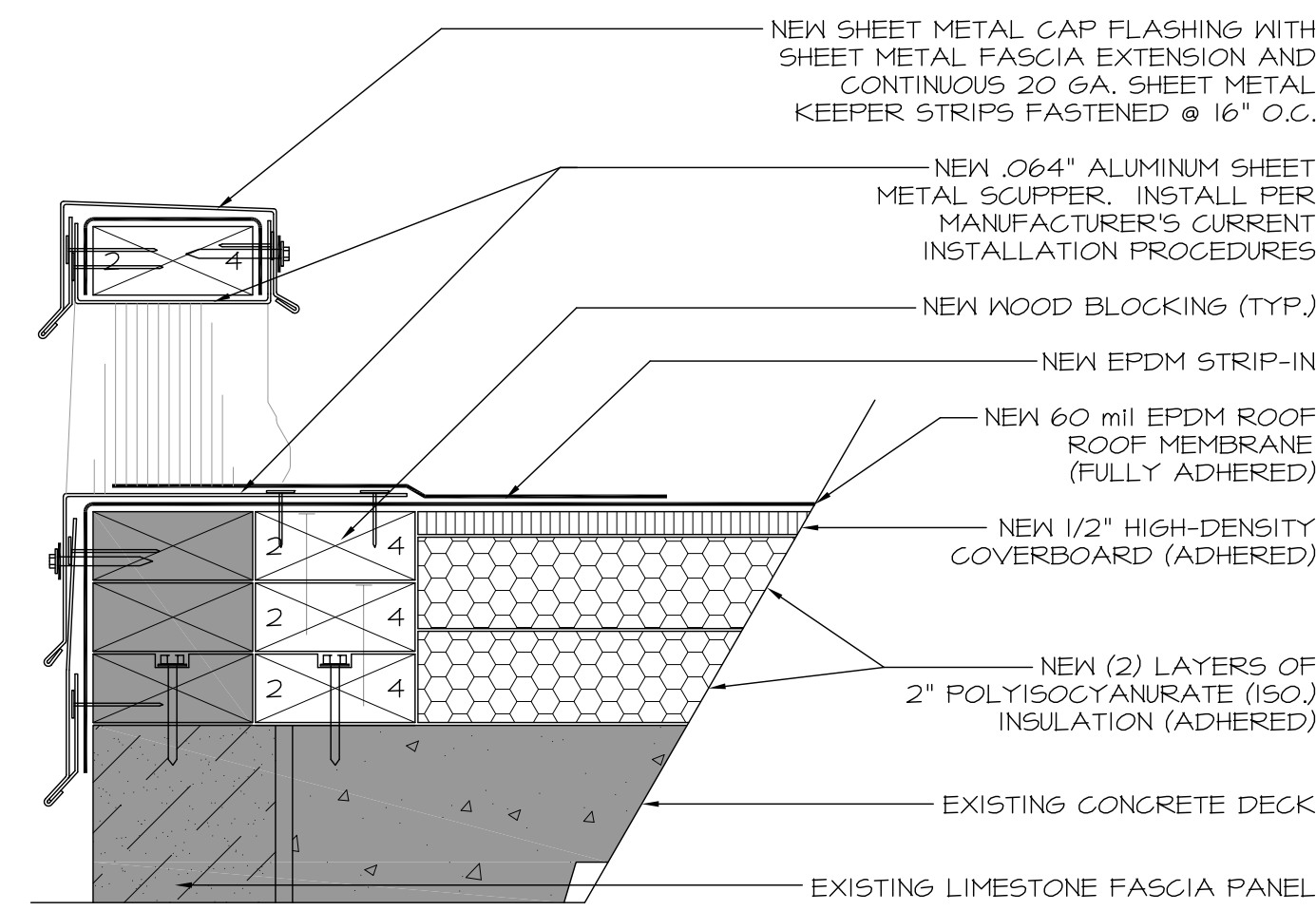
2 OVERFLOW SCUPPER FLASHING SCALE: 3"=1'-0"
