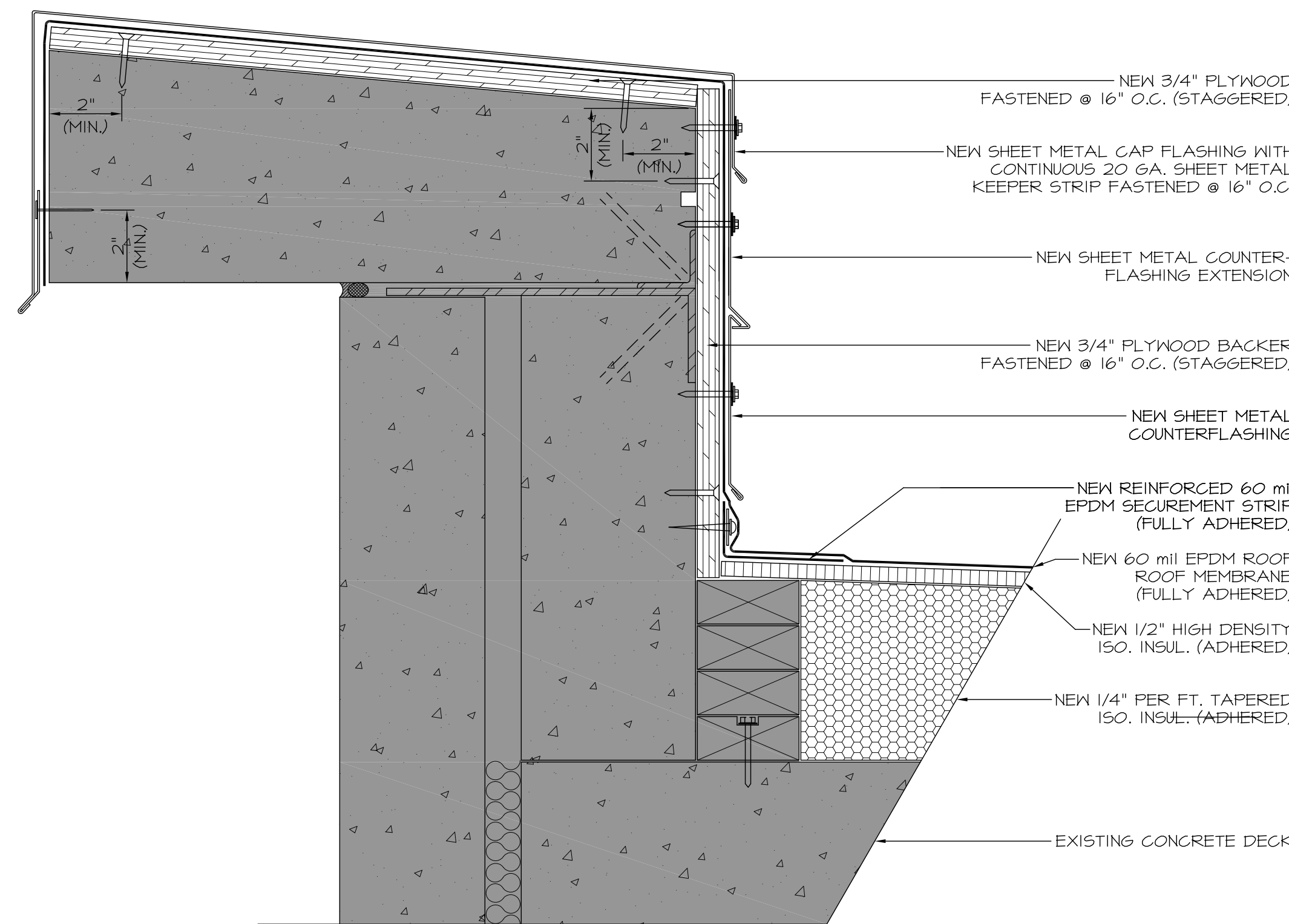
2 PARAPET FLASHING DETAIL SCALE: 3"=1'-0"
