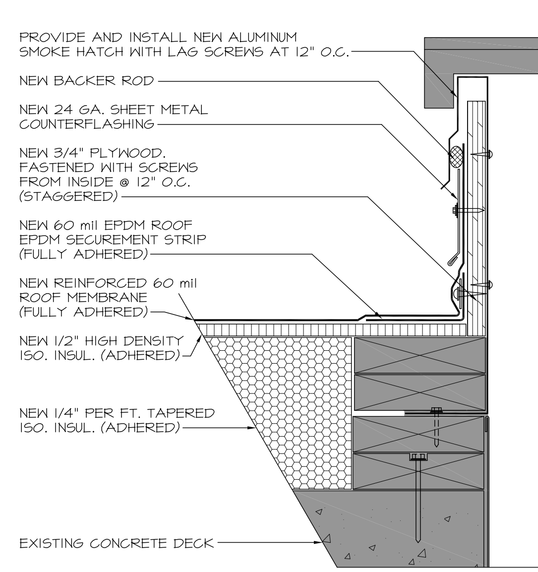
5 SMOKE HATCH DETAIL 2 SCALE: 3"=1'-0"
