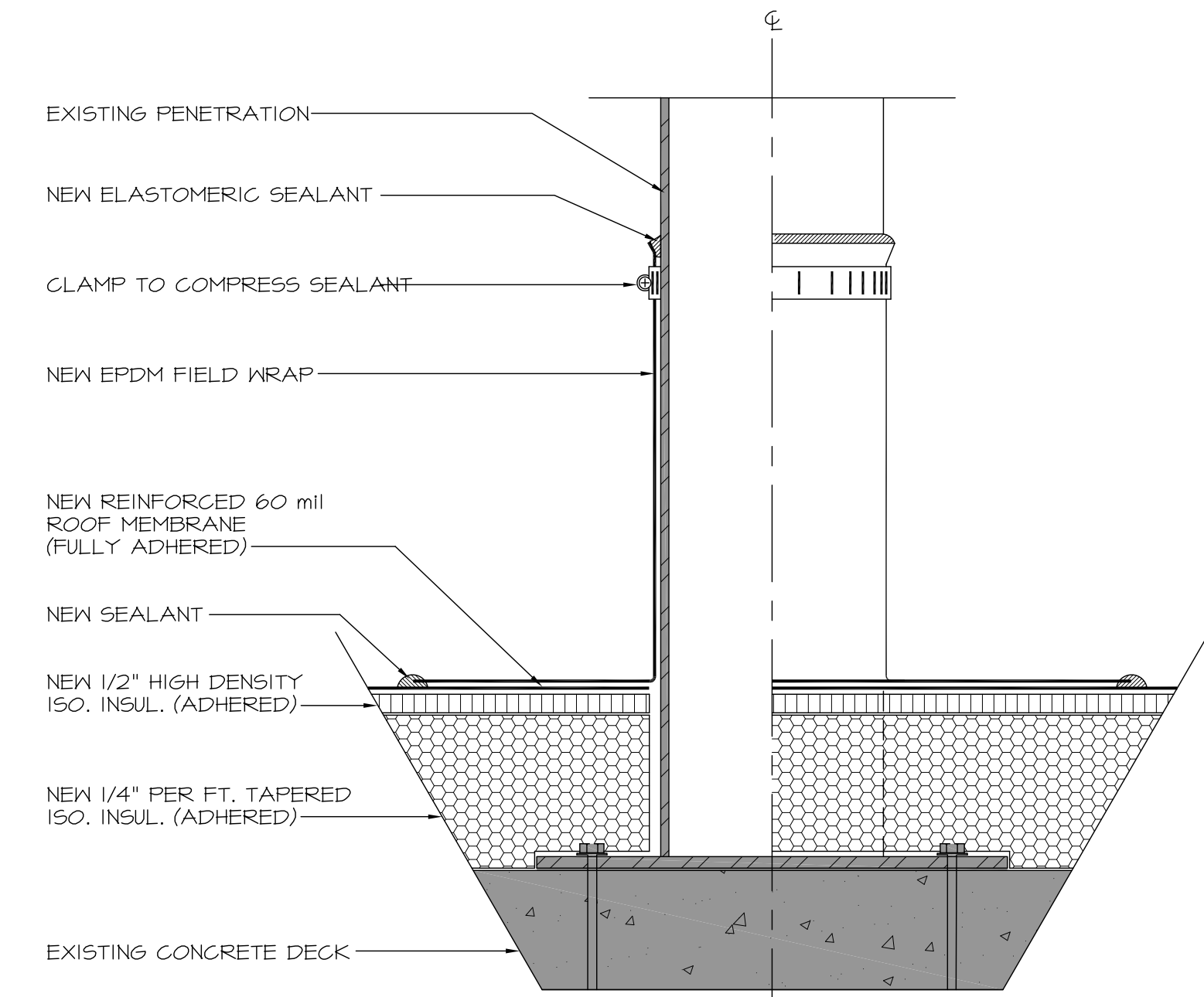
7 DAVIT FLASHING DETAIL 2 SCALE: 3"=1'-0"
