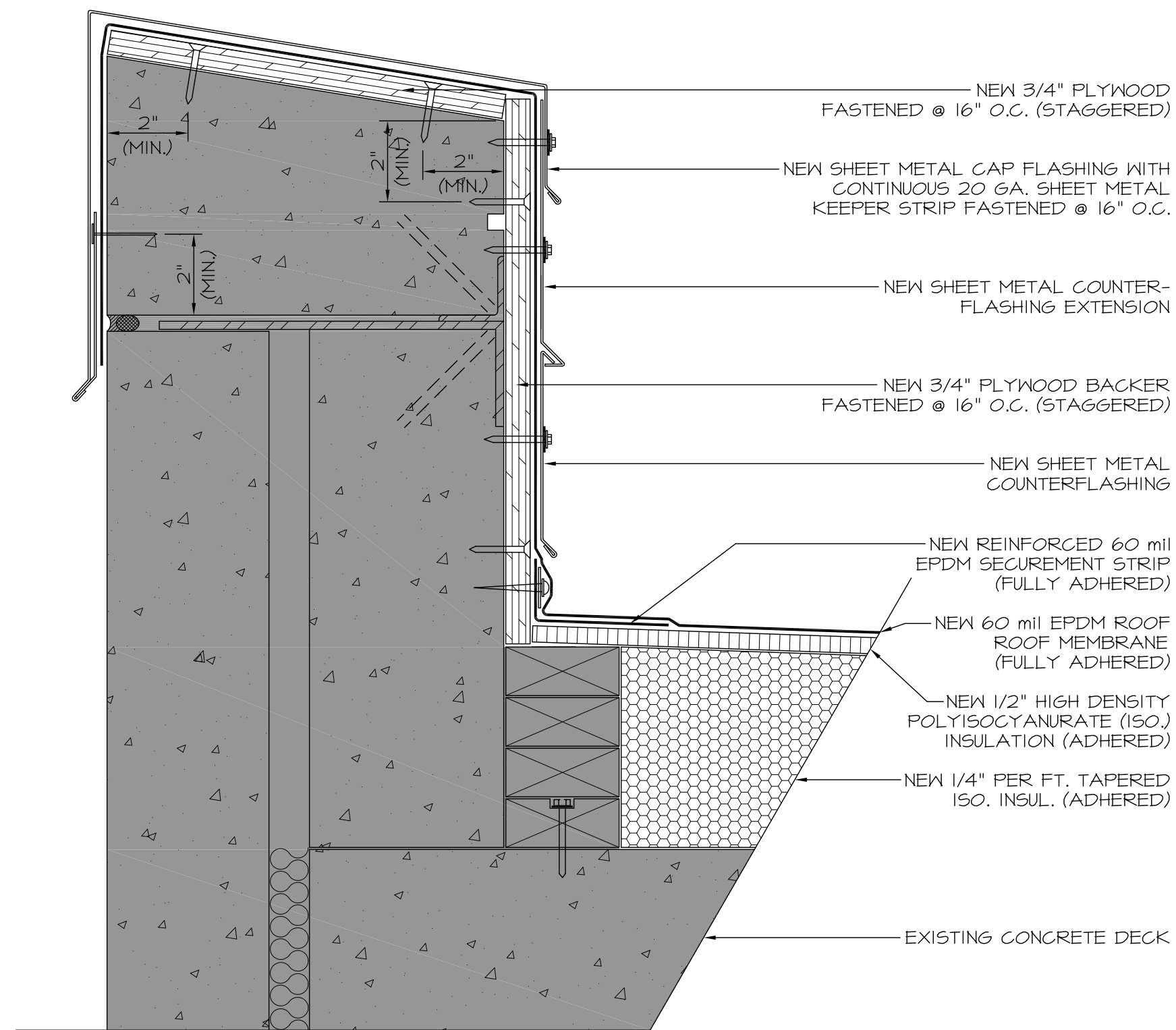
1 PARAPET FLASHING DETAIL SCALE: 3"=1'-0"
