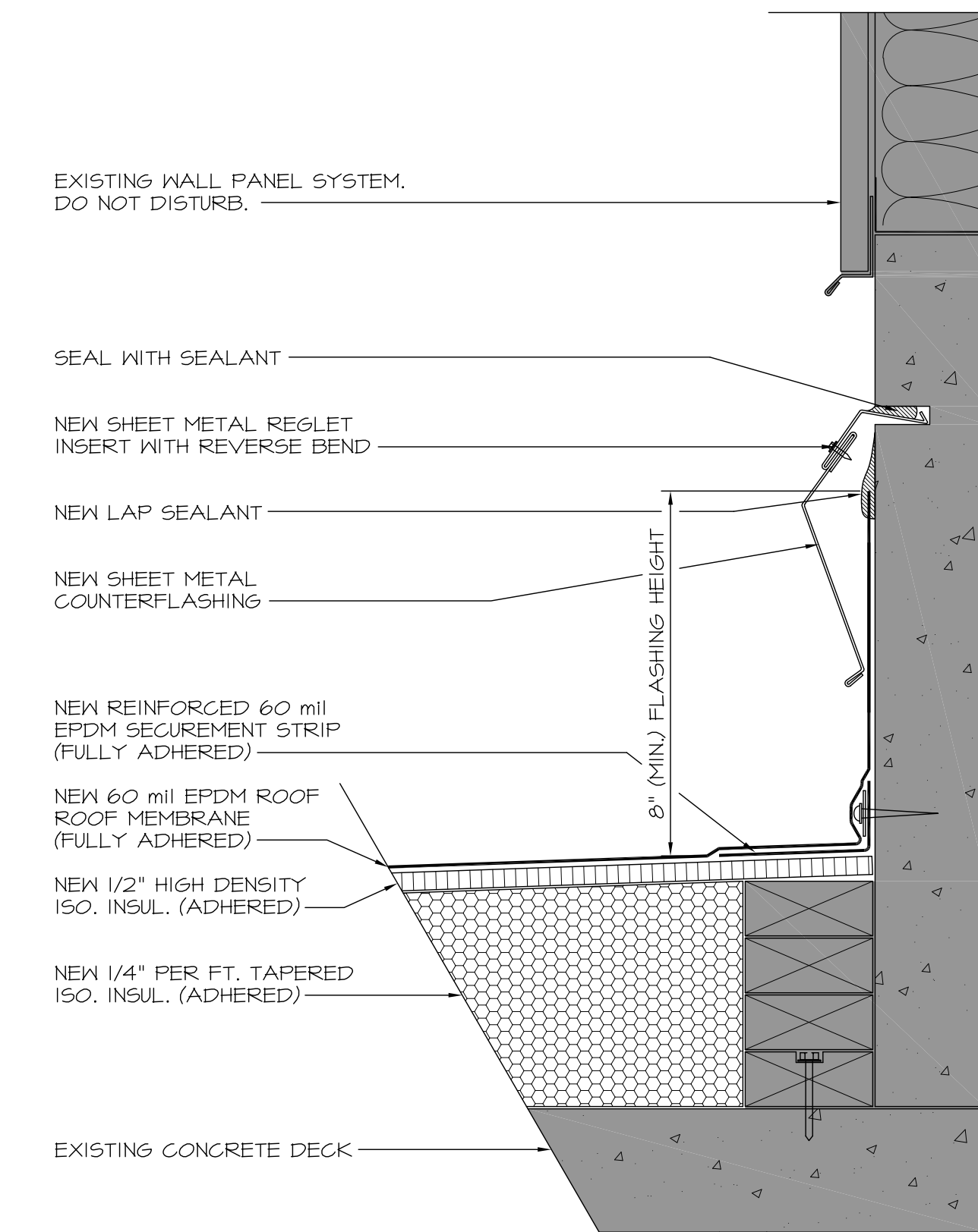
3 WALL FLASHING DETAIL SCALE: 3"=1'-0"
