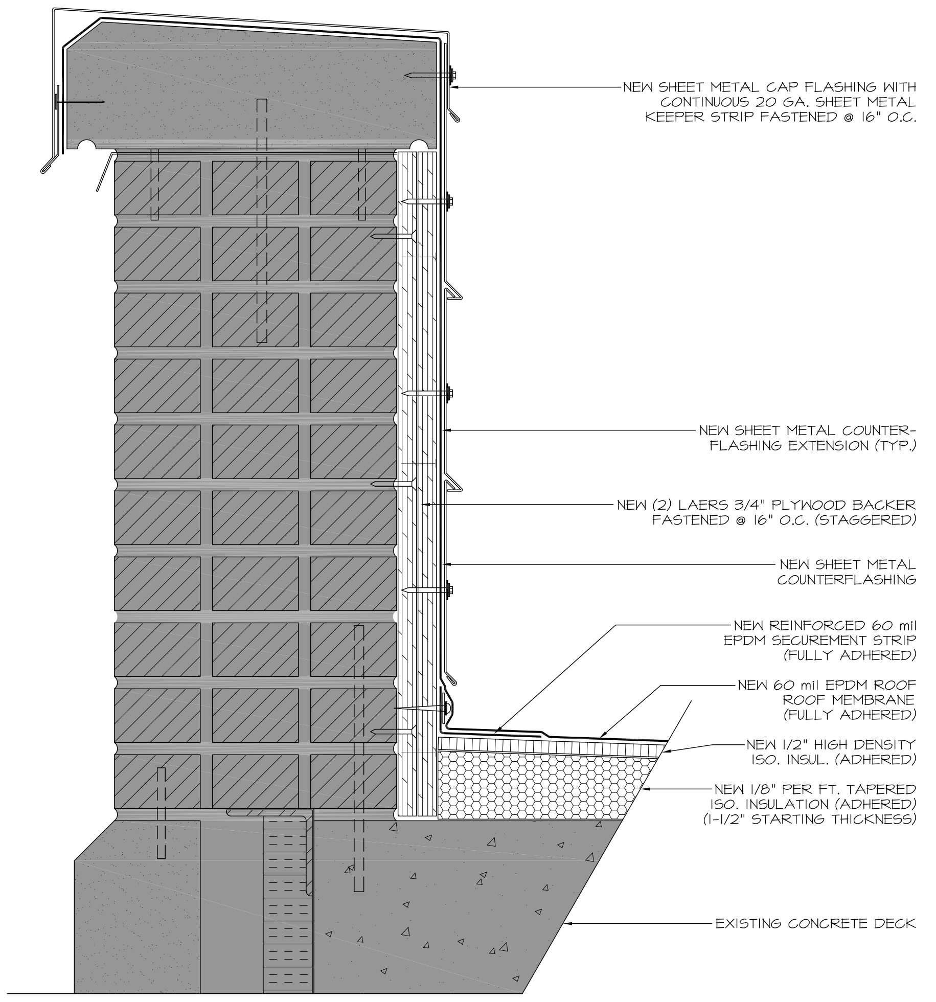
2 1 PARAPET FLASHING DETAIL SCALE: 3"=1'-0"
