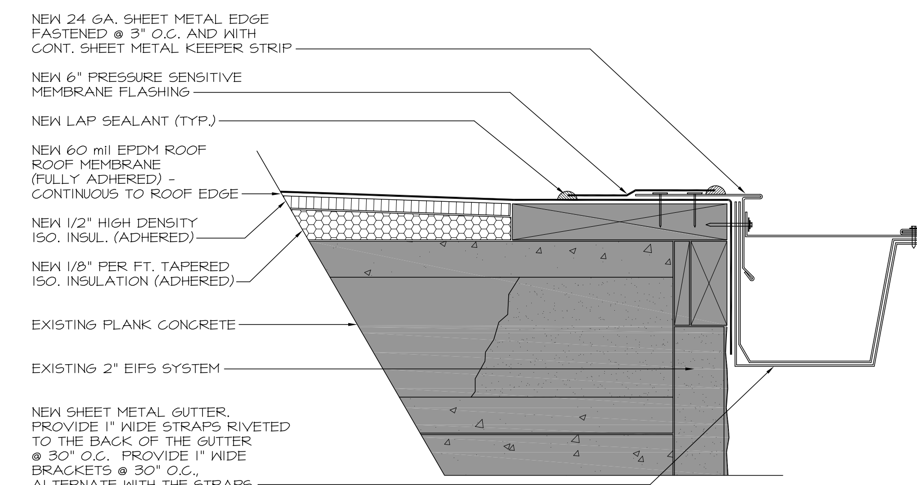
8 GUTTER EDGE FLASHING 2 SCALE: 3"=1'-0"
