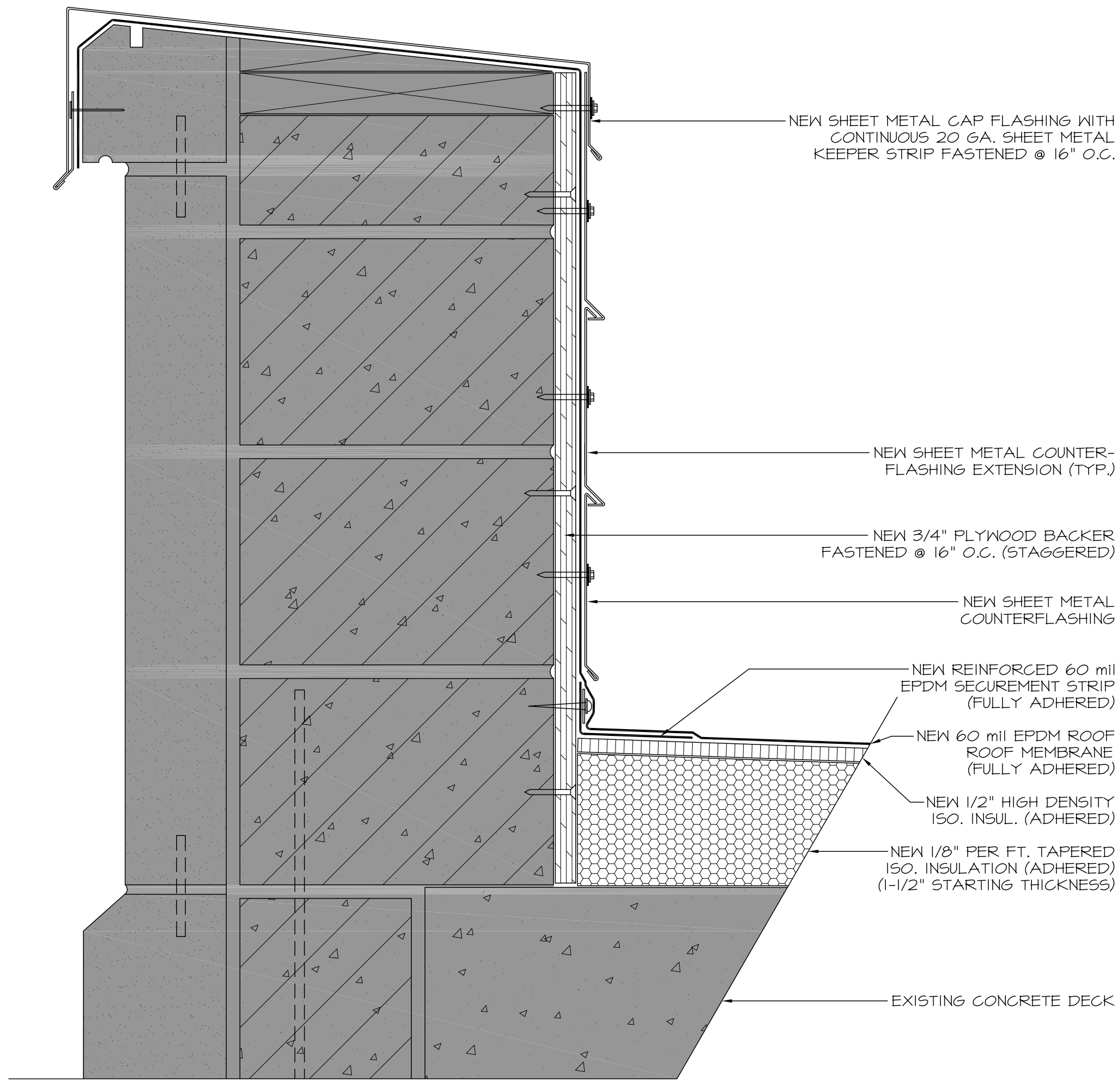
4 PARAPET FLASHING DETAIL 2 SCALE: 3"=1'-0"
