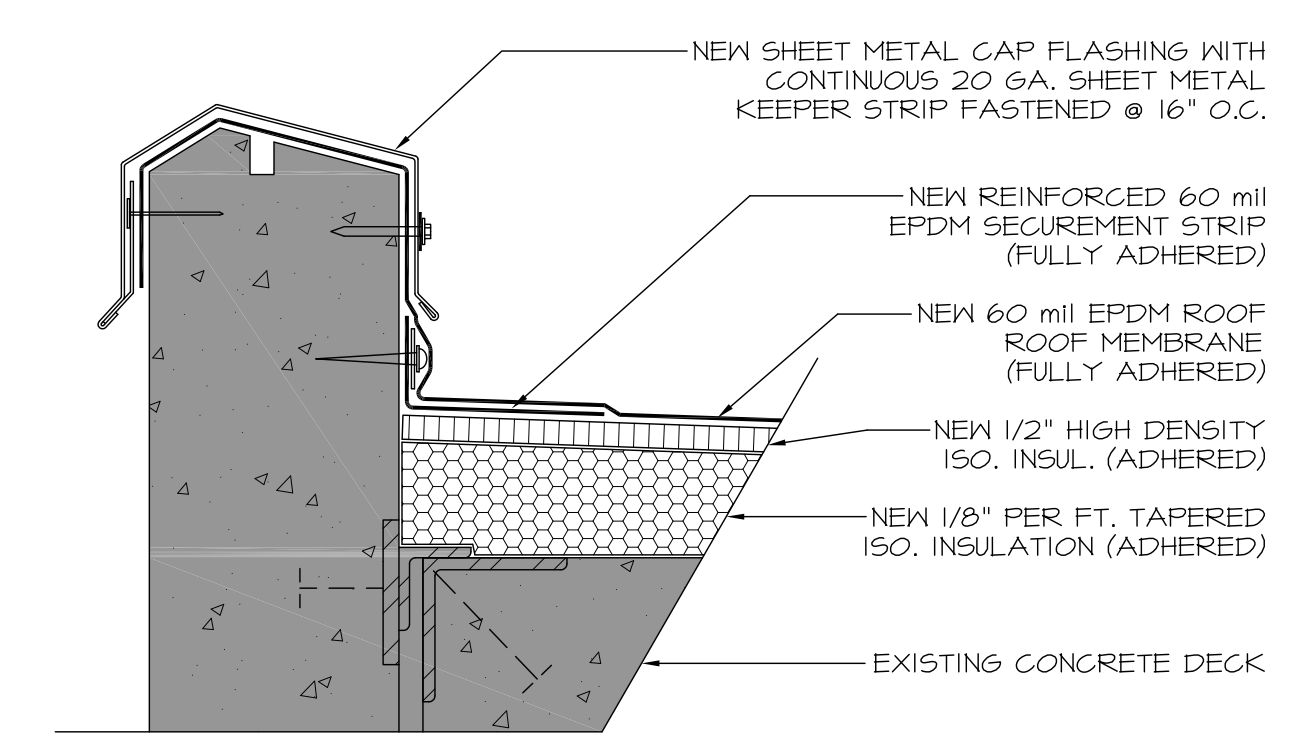
9 CANOPY PARAPET FLASHING 2 SCALE: 3"=1'-0"
