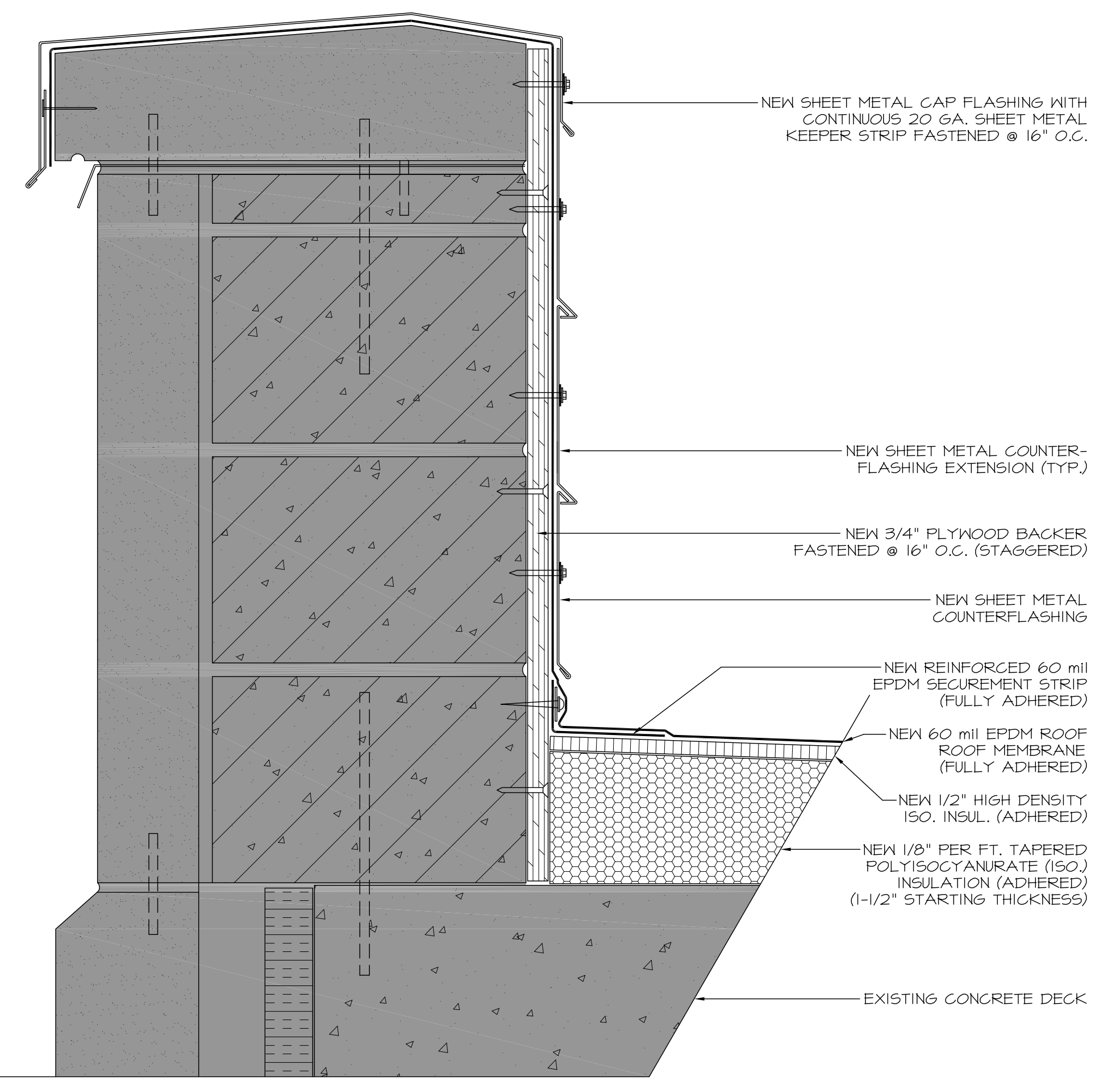
1 1 PARAPET FLASHING DETAIL SCALE: 3"=1'-0"
