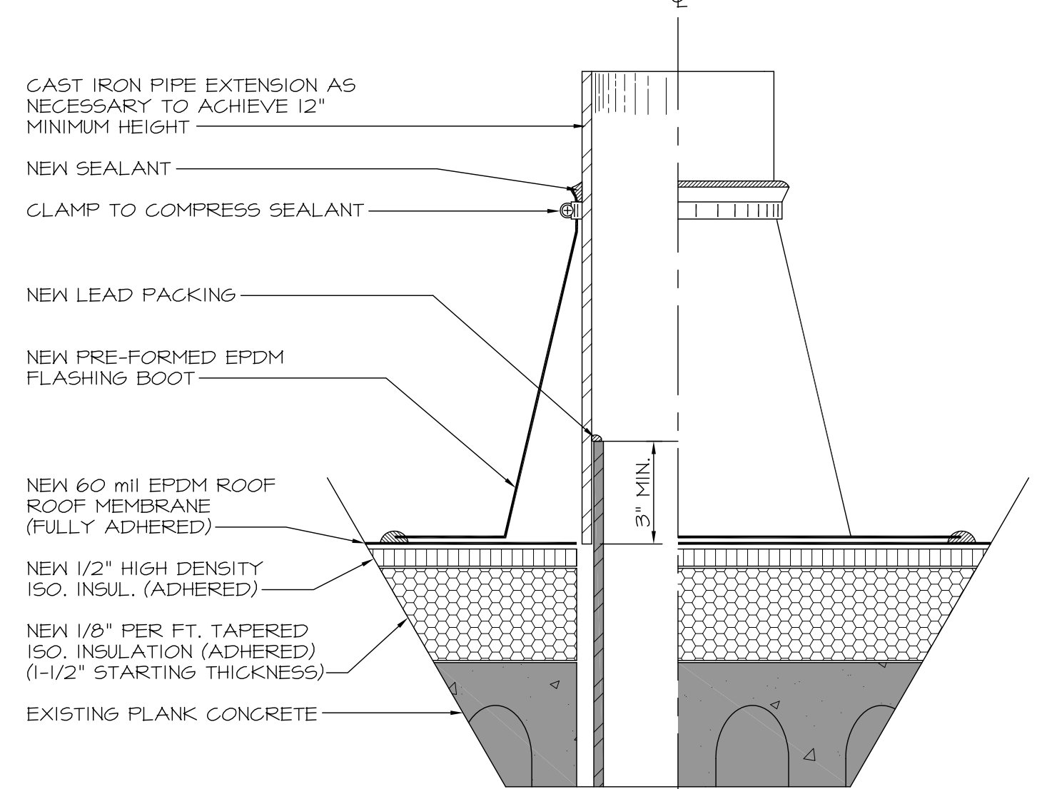
17 PLUMBING VENT DETAIL 3 SCALE: 3"=1'-0"
