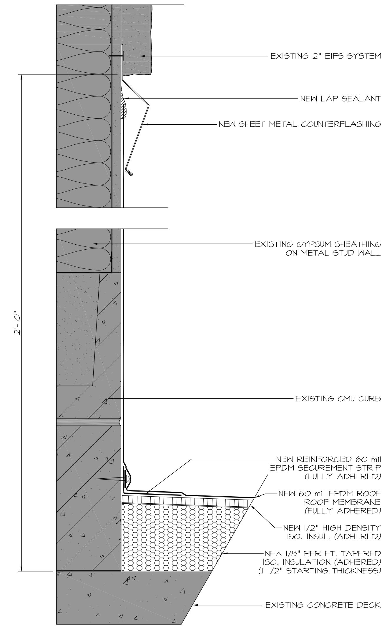
5 WALL FLASHING DETAIL 2 SCALE: 3"=1'-0"
