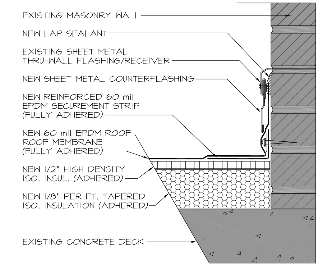
10 WALL FLASHING DETAIL 2 SCALE: 3"=1'-0"
