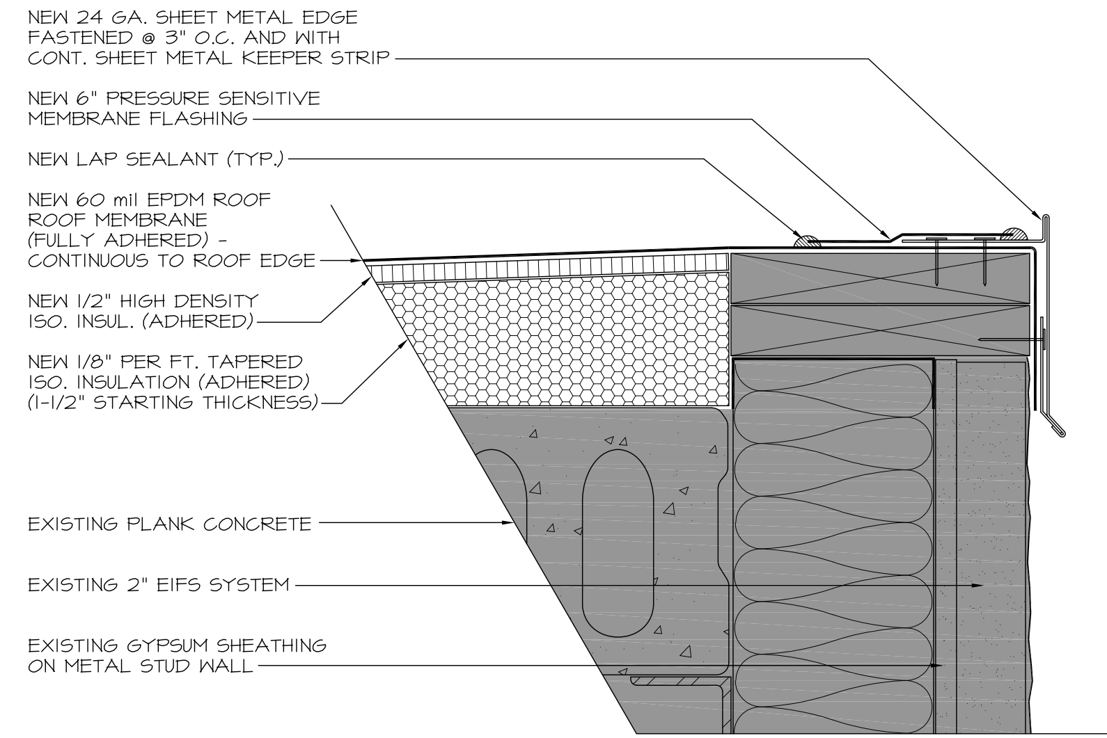
7 EDGE FLASHING DETAIL 2 SCALE: 3"=1'-0"
