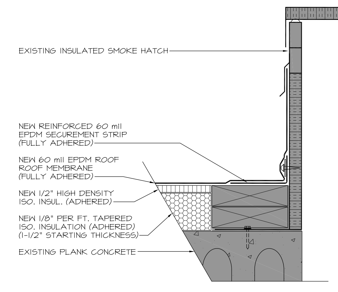
14 SMOKE HATCH DETAIL 3 SCALE: 3"=1'-0"
