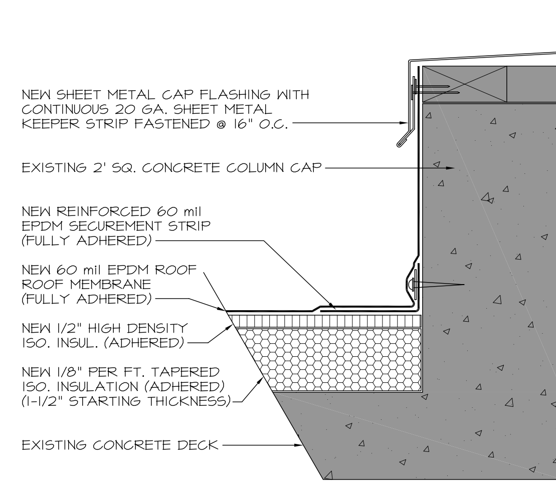
12 COLUMN CAP FLASHING DETAIL 3 SCALE: 3"=1'-0"
