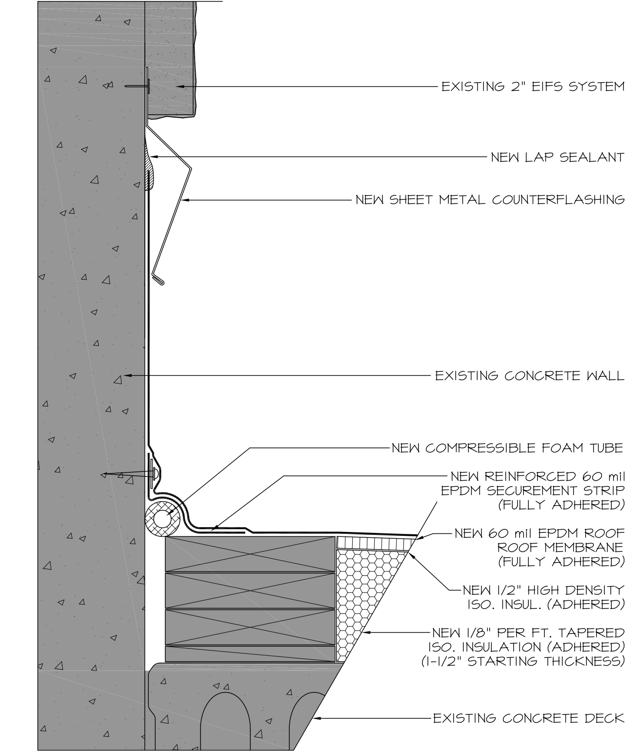
6 WALL FLASHING DETAIL 2 SCALE: 3"=1'-0"
