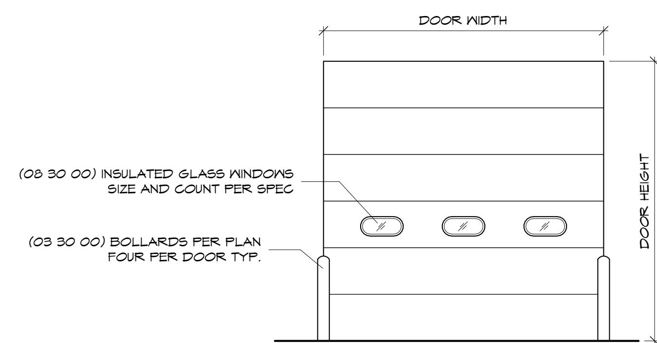
Typ OH Door
