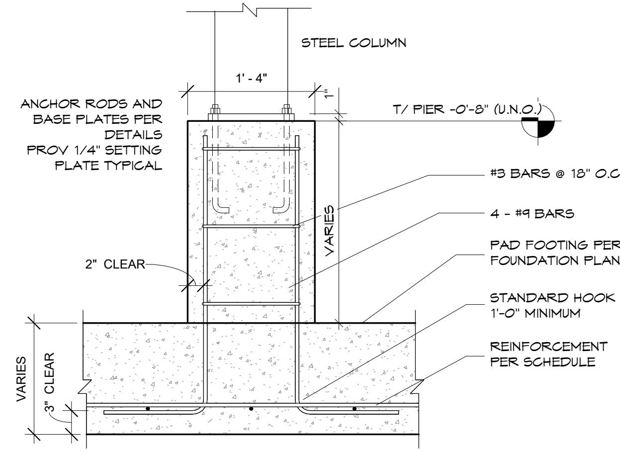
8 Pier - Typ 1" = 1'-0"
