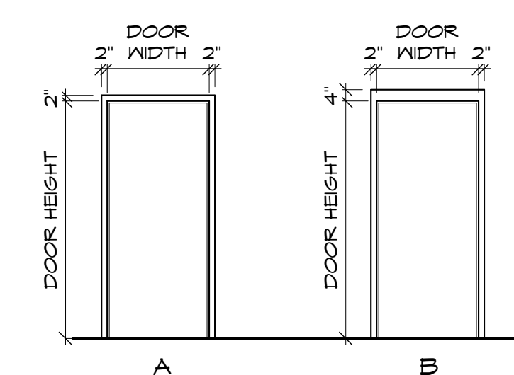
Door Frame Types
